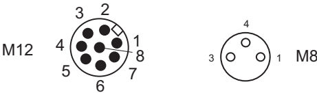
接头 /Joint
